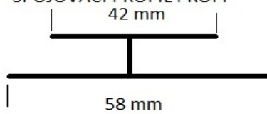
SPOJOVACÍ PROFIL PROFI
