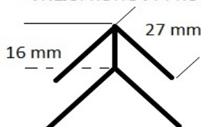
VNĚJŠÍ ROHOVÝ PROFIL
